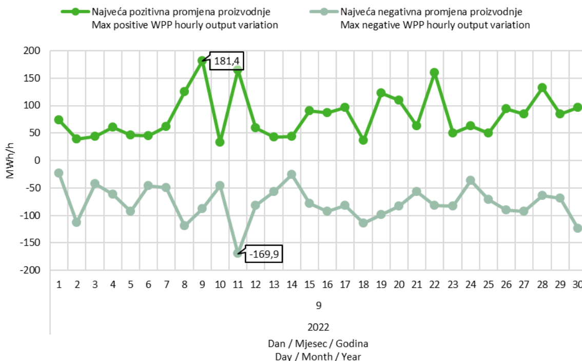
Slika 9 Maksimalna pozitivna i maksimalna negativna promjena satne proizvodnje VE u rujnu 2022. godine
