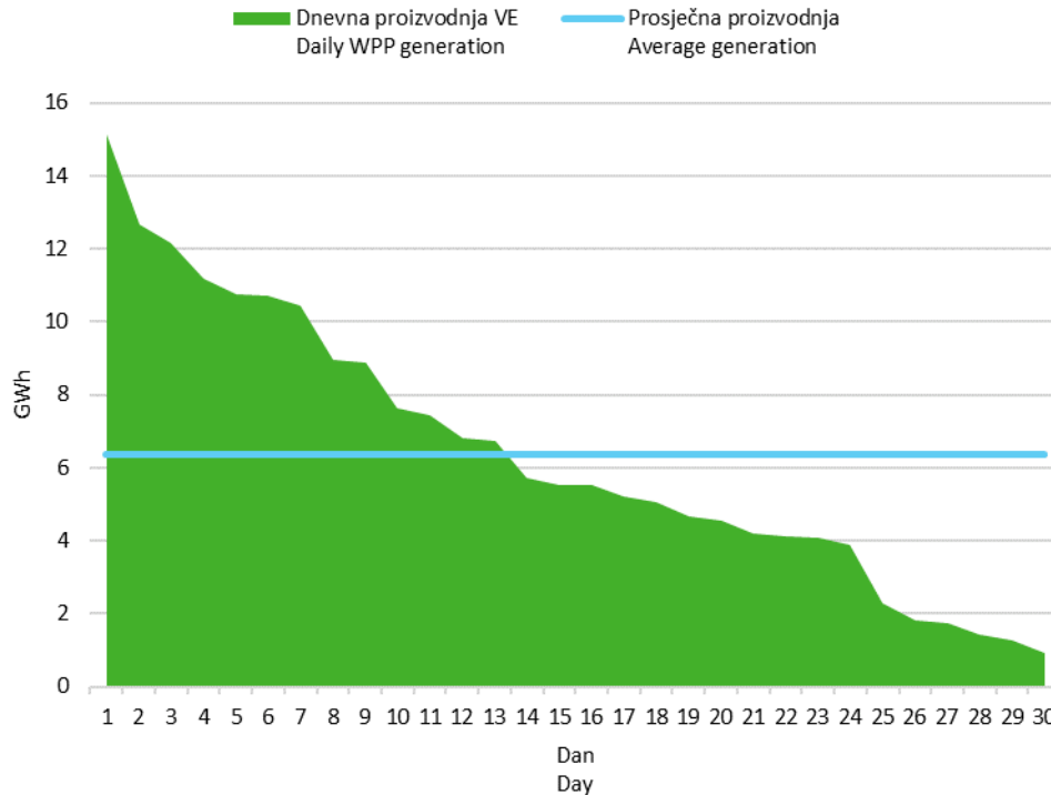
Slika 6 Krivulja trajanja dnevne proizvodnje vjetroelektrana u rujnu 2022. godine
