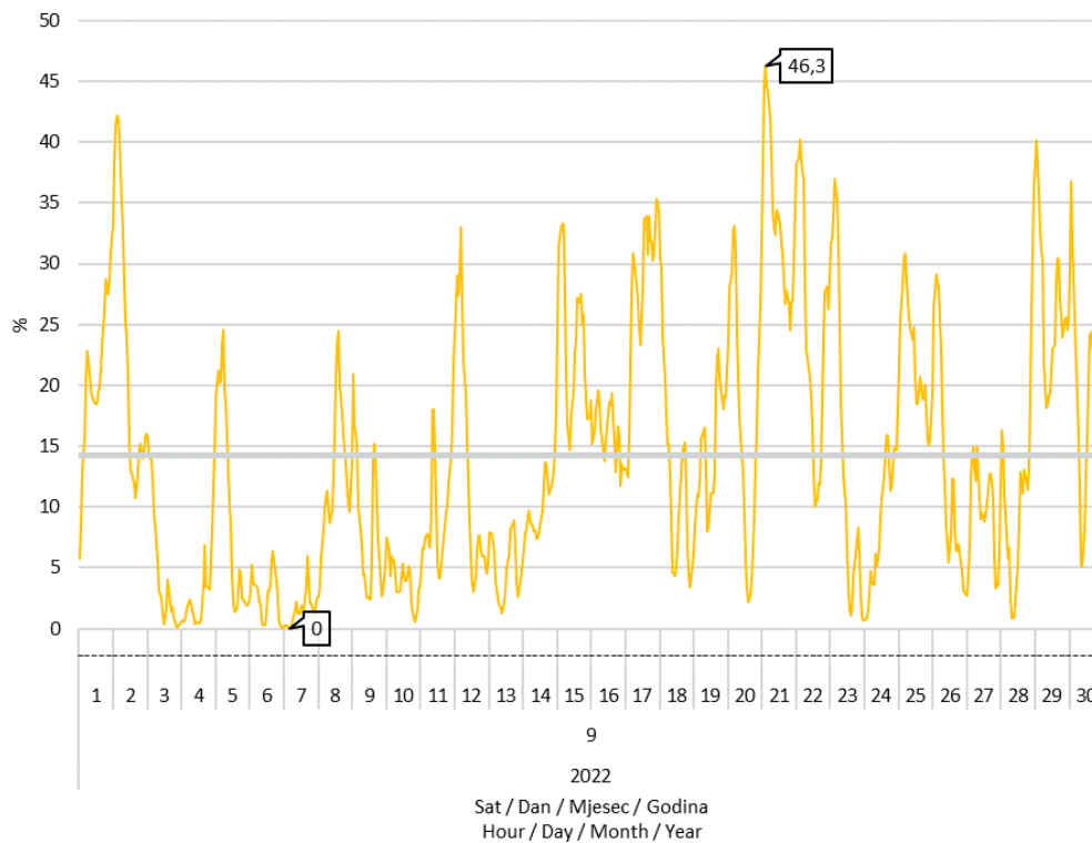
Slika 8 Udio proizvodnje vjetroelektrana u pokrivanju satnog opterećenja elektroenergetskog sustava u rujnu 2022. godine
