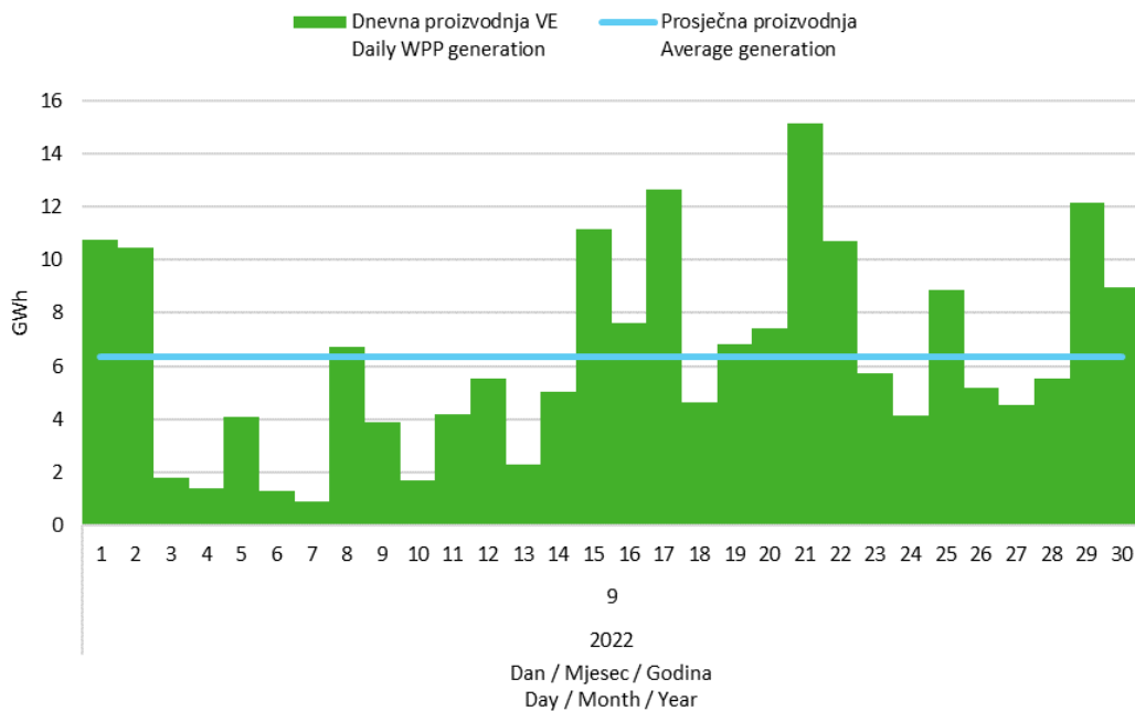
Slika 5 Dnevna proizvodnja svih vjetroelektrana u rujnu 2022. godine Figure 5 Daily generation of all wind power plants in September 2022
