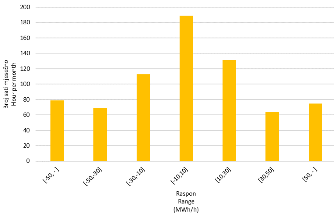
Slika 10 Statistička raspodjela satnih promjena proizvodnje VE u rujnu 2022. godine Figure 10 Statistical distribution of WPP hourly output variations in September 2022
