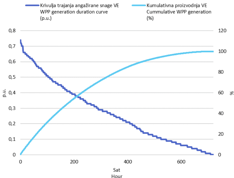
Slika 3 Krivulja trajanja angažirane snage svih VE i kumulativna proizvodnja VE u rujnu 2022. godine u jediničnim vrijednostima
