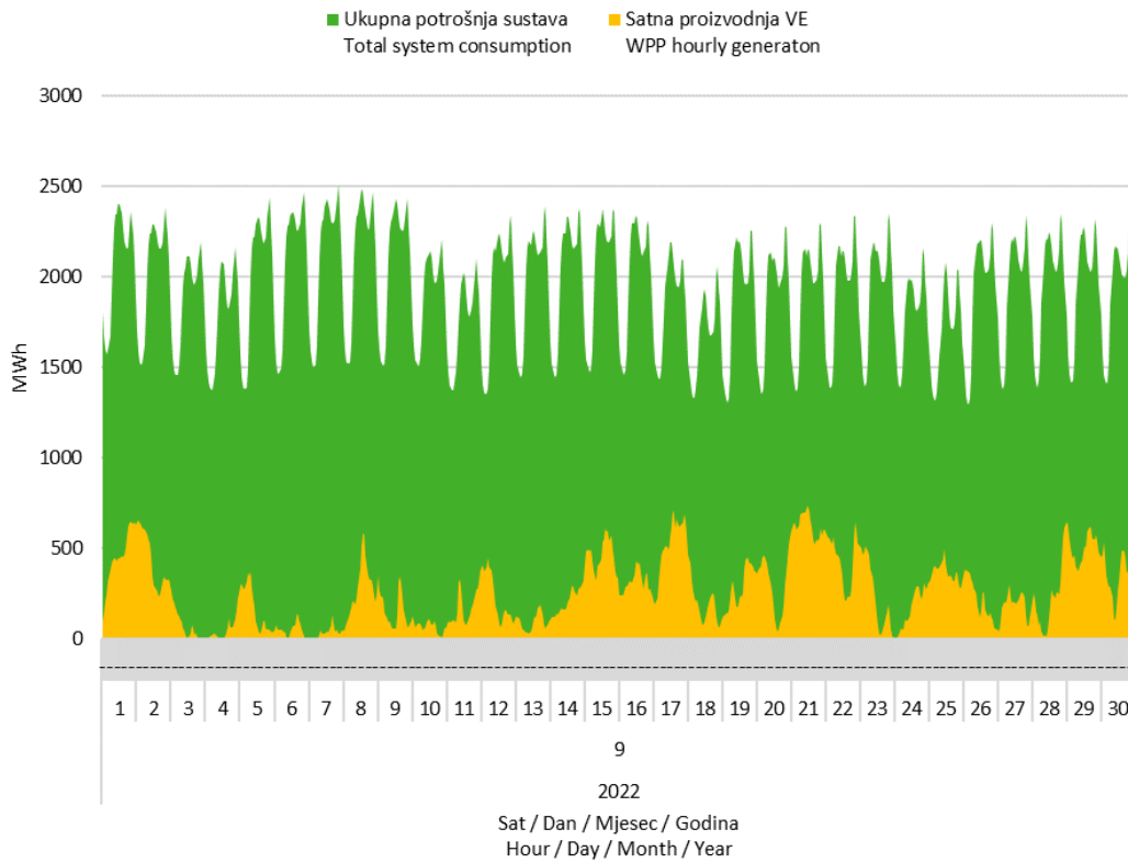
Slika 7 Usporedba satnog dijagrama opterećenja sustava i proizvodnje vjetroelektrana u rujnu 2022. godine
