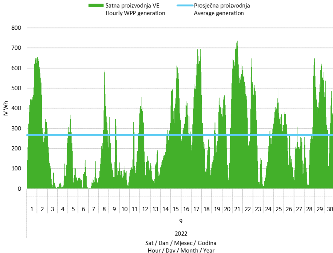
Slika 2 Satna proizvodnja svih vjetroelektrana u rujnu 2022. godine Figure 2 Hourly generation of all wind power plants in September 2022
